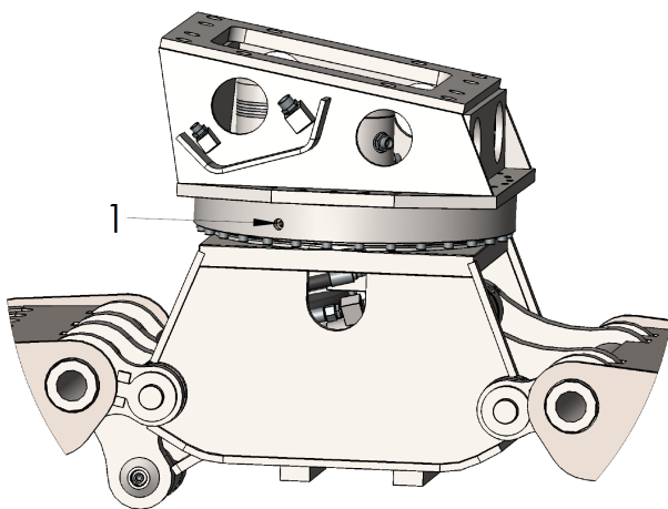
Afbeelding 5: Smering draaikrans
