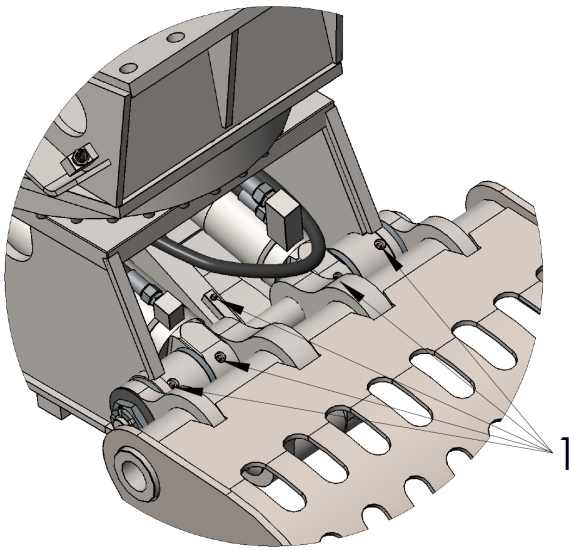
Afbeelding 3: Smering draaipunten
