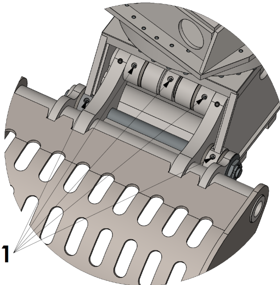
Afbeelding 4: Smering draaipunten
