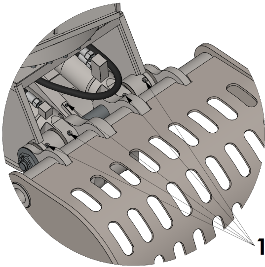
Afbeelding 3: Smering draaipunten
