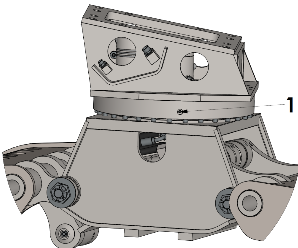
Afbeelding 5: Smering draaikrans
