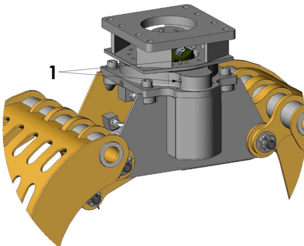
Afbeelding 5: Smering Draaikrans
